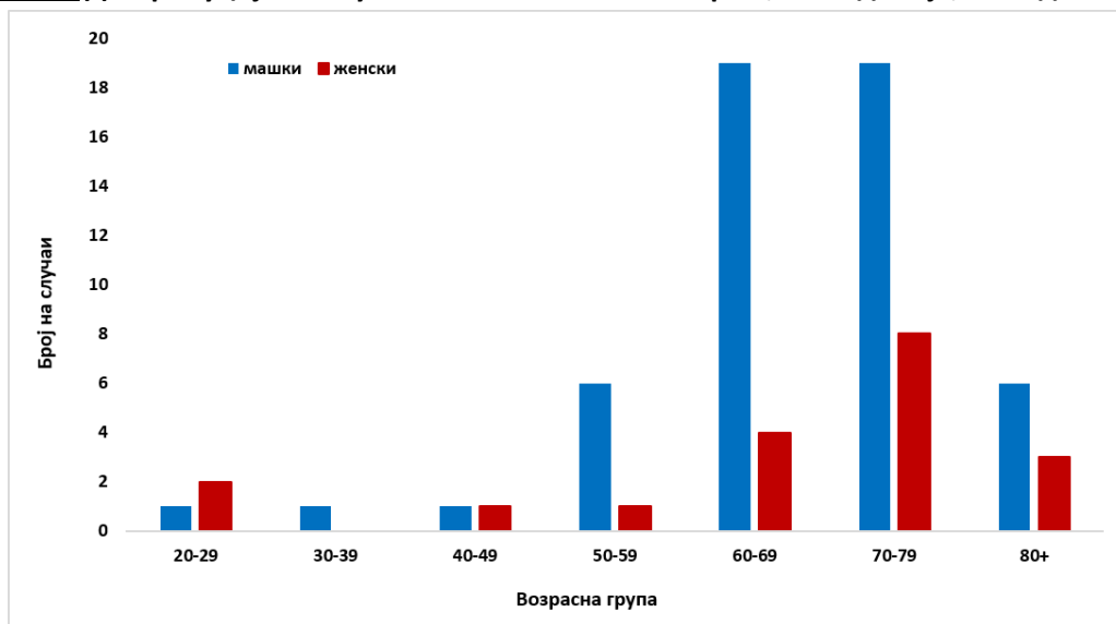
Графикон 1. Дистрибуција на случаи на WNV по пол и возраст, Македонија, 2026 до 27.10.2026
