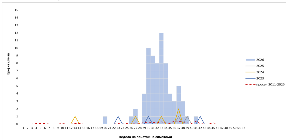
Графикон 2. Број на пријавени случаи на WNV по недела на појава на симптоми, Македонија, 2023, 2024, 2025, просек 2011-2025, 2026 до 27.10.2026
